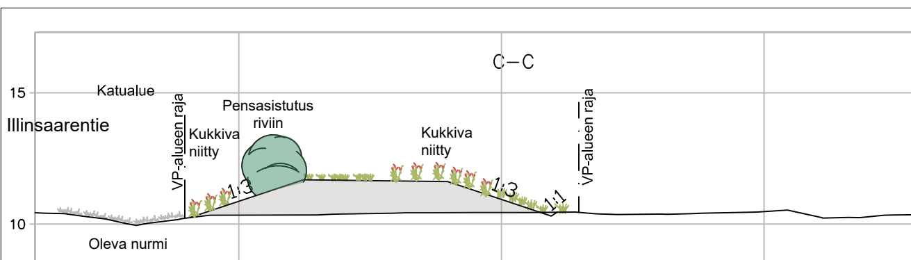
POIKKILEIKKAUS 1:200 B - B
