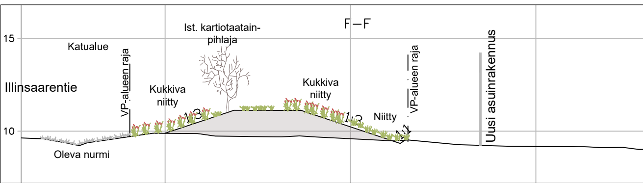
POIKKILEIKKAUS 1:200 E - E
