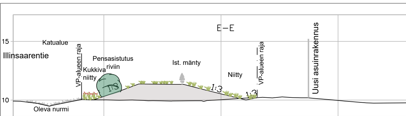
POIKKILEIKKAUS 1:200 D - D
