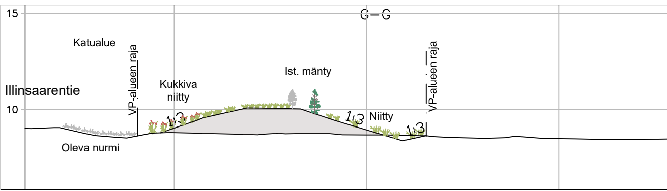
POIKKILEIKKAUS 1:200 F - F
