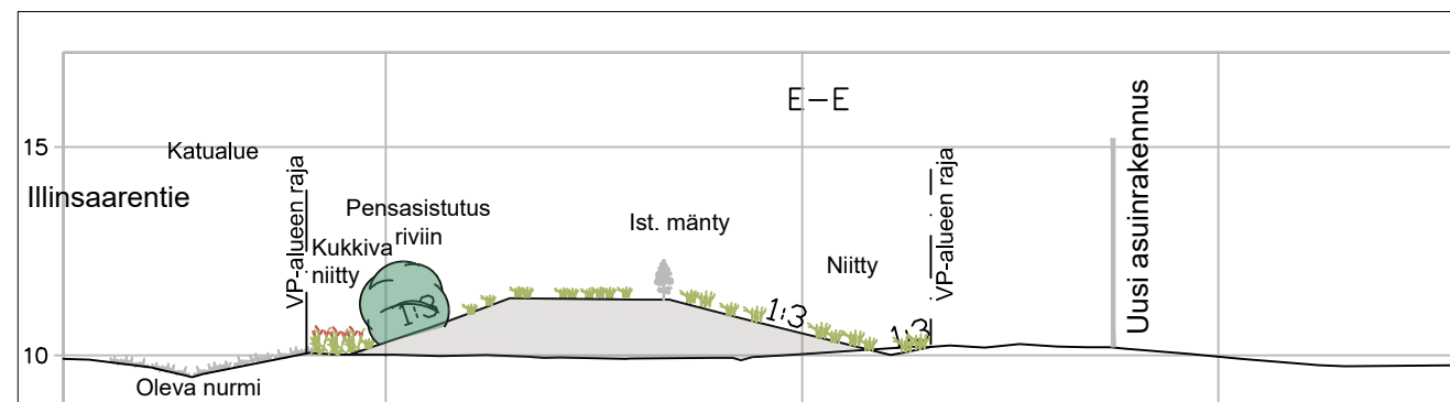
POIKKILEIKKAUS 1:200 D - D
