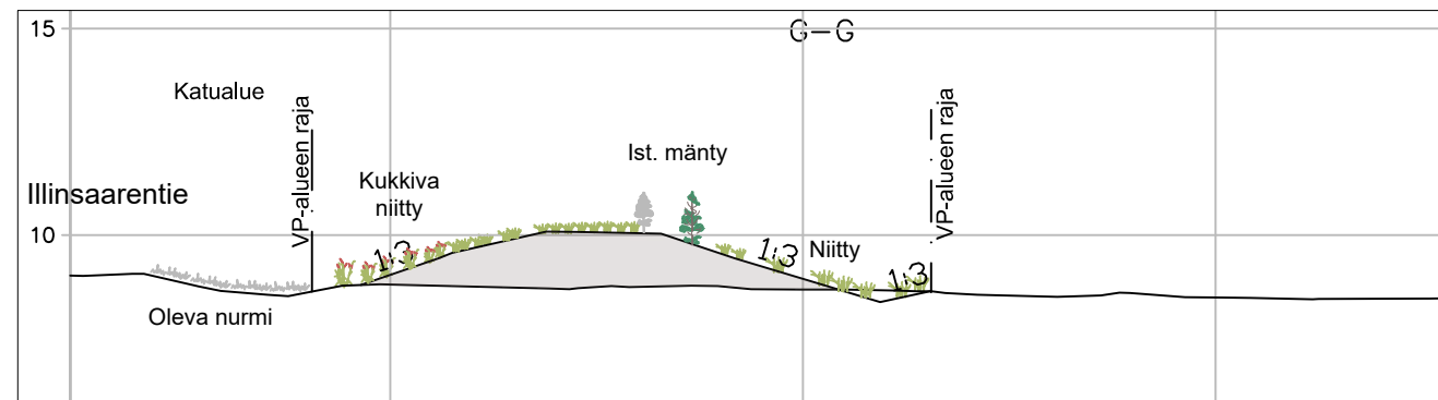
POIKKILEIKKAUS 1:200 F - F
