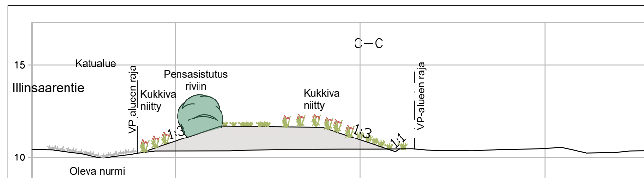
POIKKILEIKKAUS 1:200 B - B
