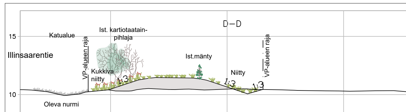
POIKKILEIKKAUS 1:200 C - C
