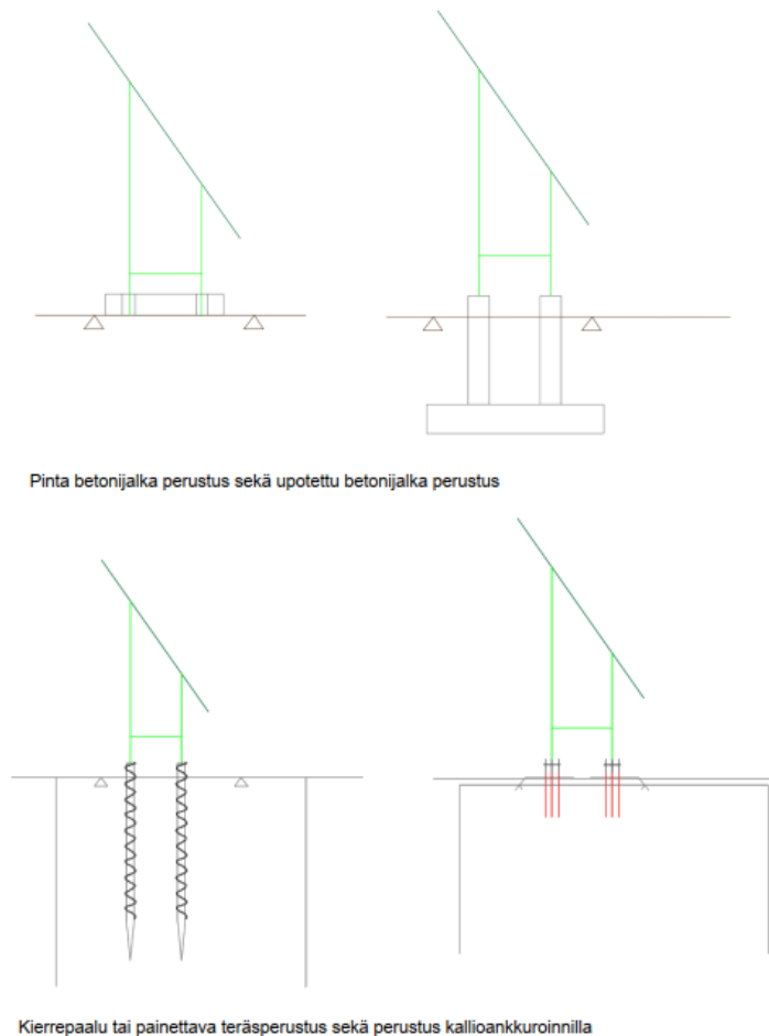
Kuva 26: Aurinkopaneelien perustustapojen periaatteita. Lähde: A-insinöörit
