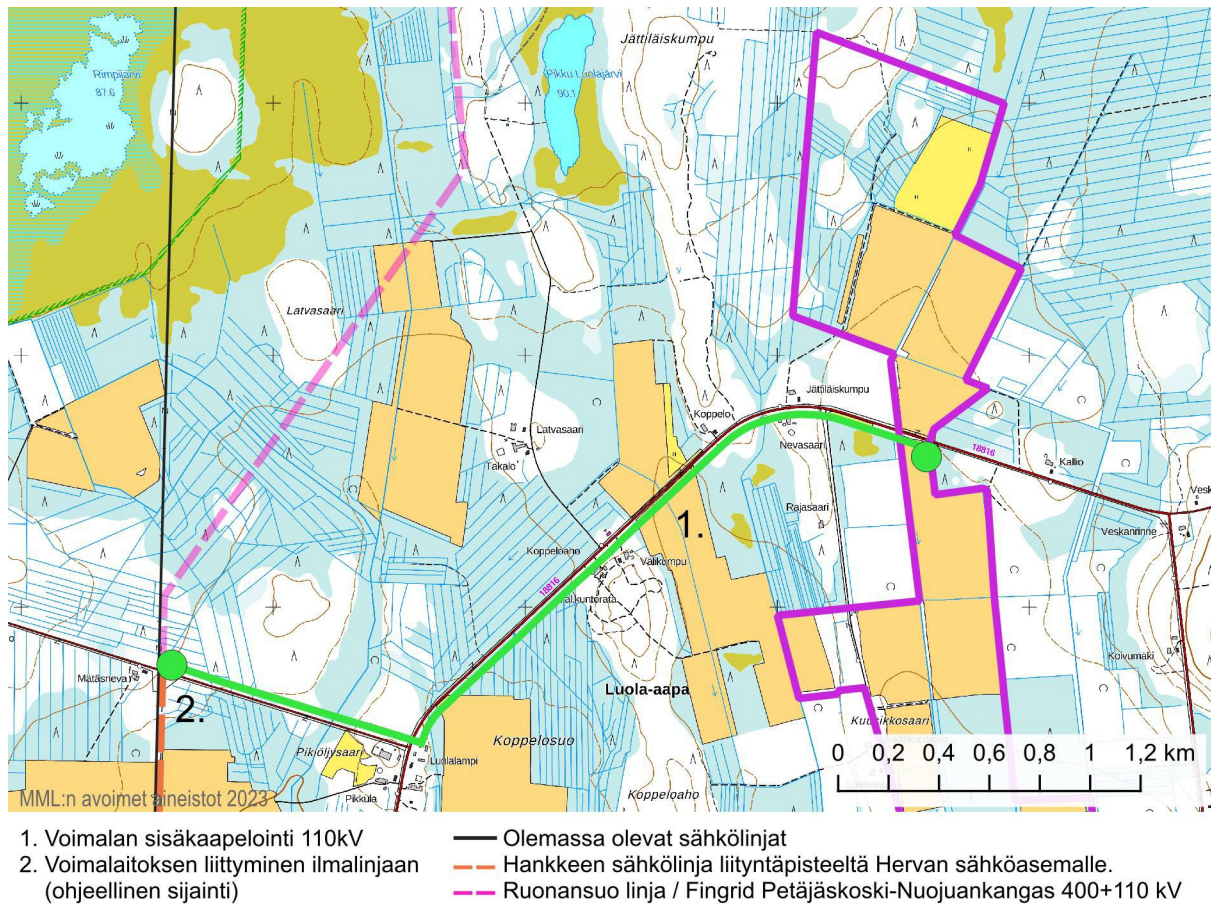
Kuva 19: Hankkeen liittyminen sähköverkkoon (Kuva: Arkkitehtitoimisto AJAK Oy).
