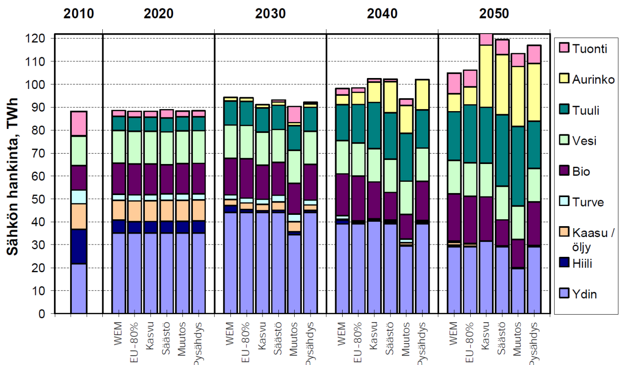
Kuva 15: Sähköenergian hankinta energialähteittäin eri skenaarioissa 2050-luvulle asti, PITKO 2019
