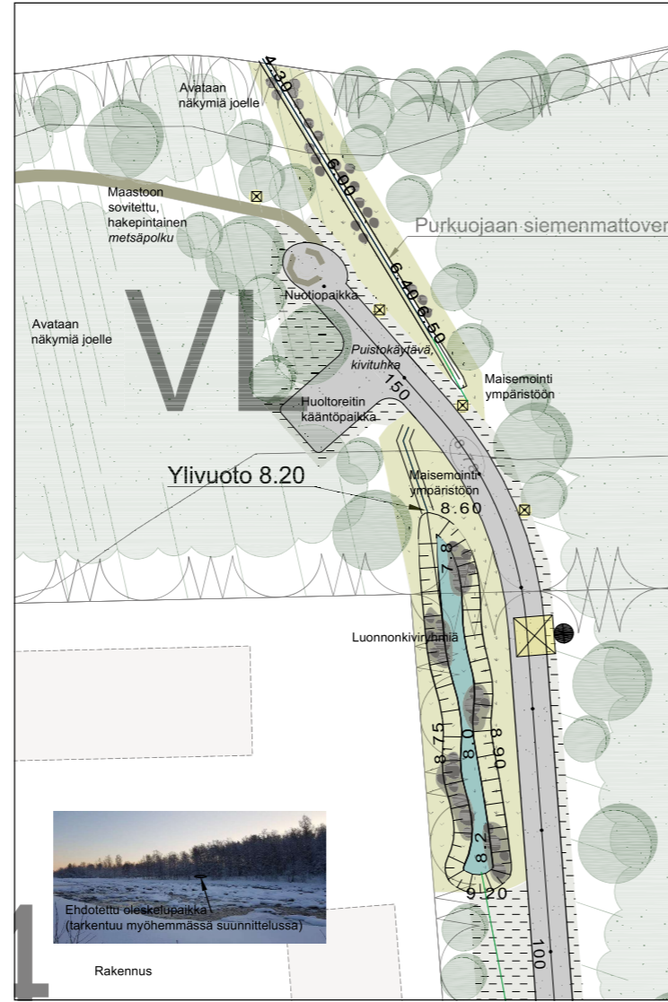
DET 1. 1:300
