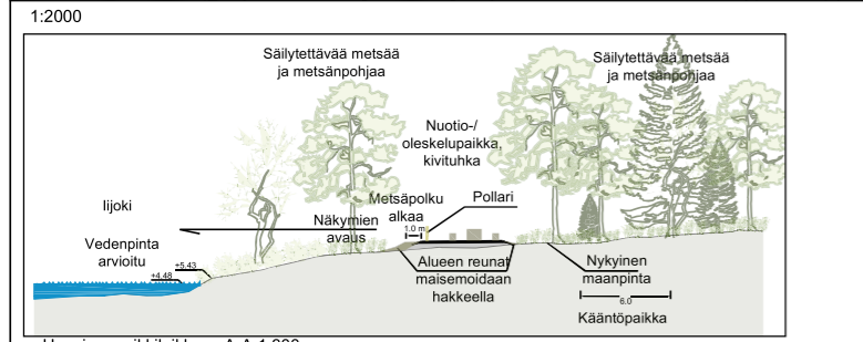
Havainnepoikkileikkaus A-A 1:300
